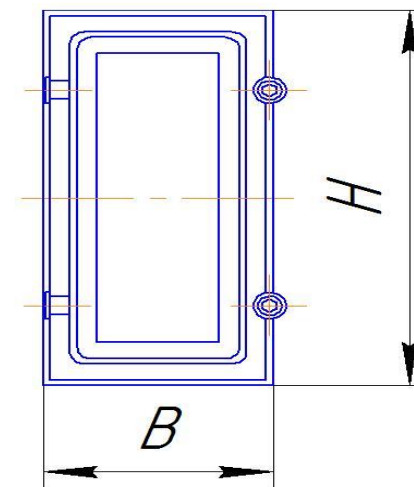
Рис. 1 Дверь герметичная для вентиляционных камер.
